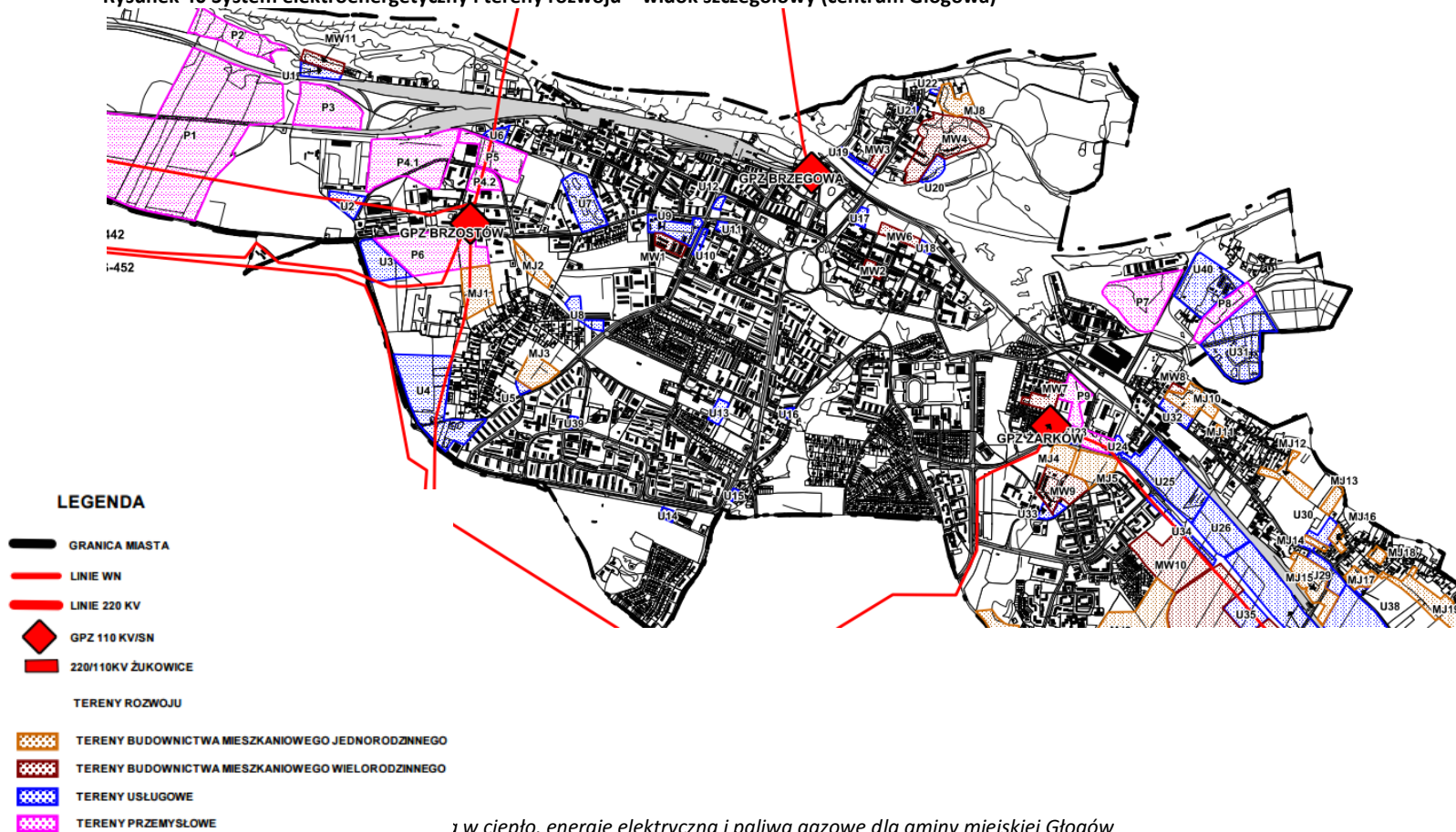
Rysunek 40 System elektroenergetyczny i tereny rozwoju – widok szczegółowy (centrum Głogowa)
