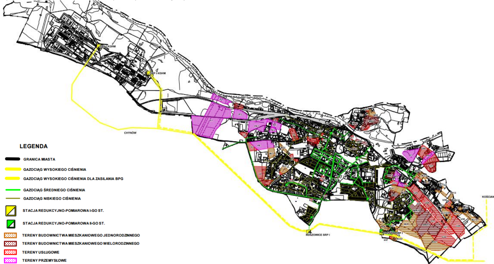
Rysunek 43 System gazowniczy i tereny rozwoju – widok ogólny
