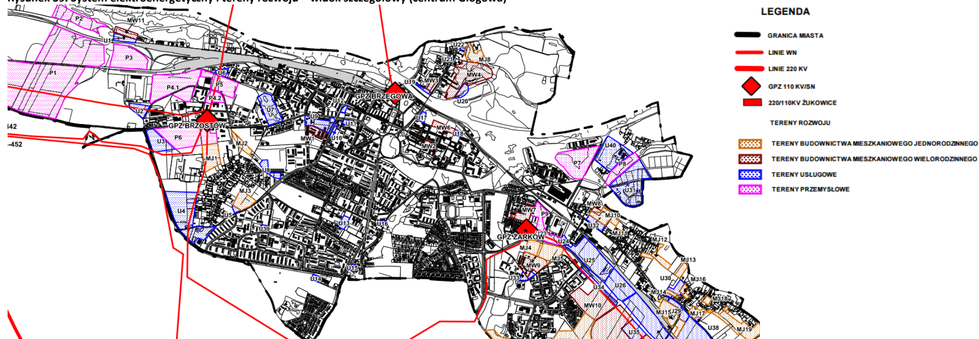
Rysunek 39. System elektroenergetyczny i tereny rozwoju – widok szczegółowy (centrum Głogowa)
