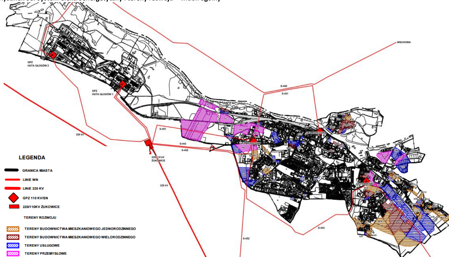
Rysunek 38. System elektroenergetyczny i tereny rozwoju – widok ogólny
