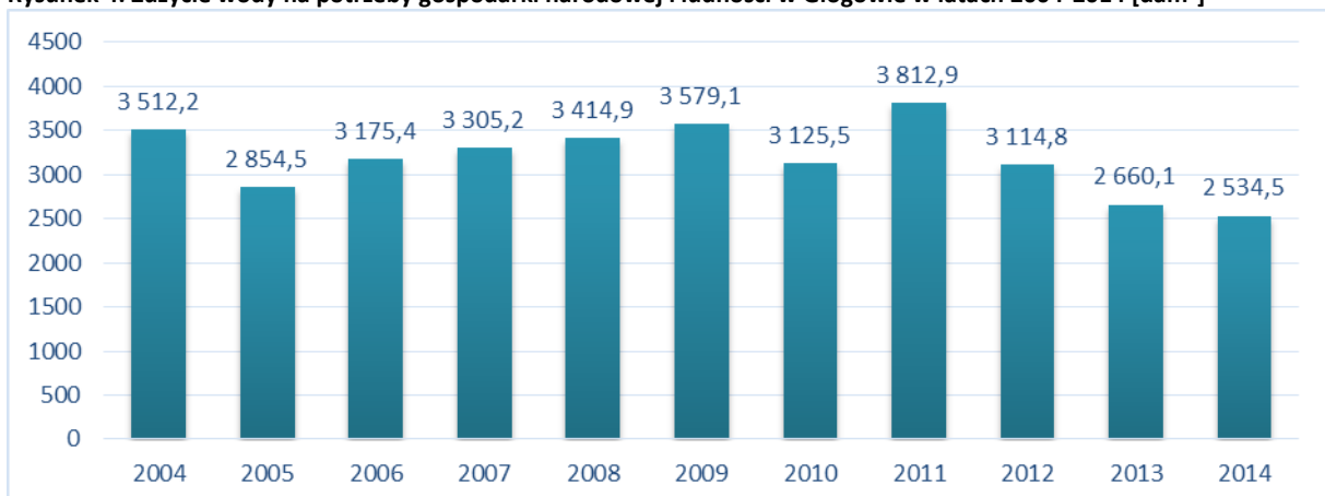
Rysunek 4. Zużycie wody na potrzeby gospodarki narodowej i ludności w Głogowie w latach 2004-2014 [dam 3 ]
